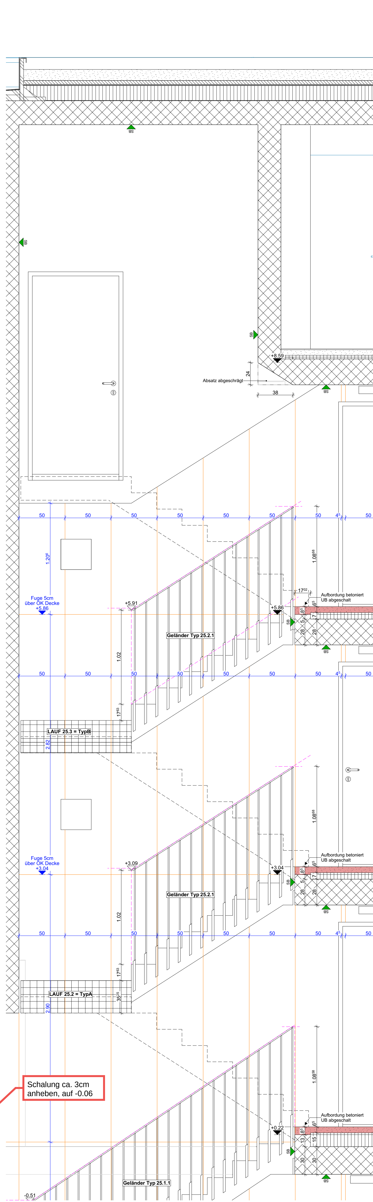
Haus 25 - Treppen Schnitt b-b
